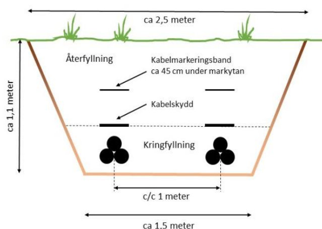
Figur 5 Exempel på schaktskiss.
